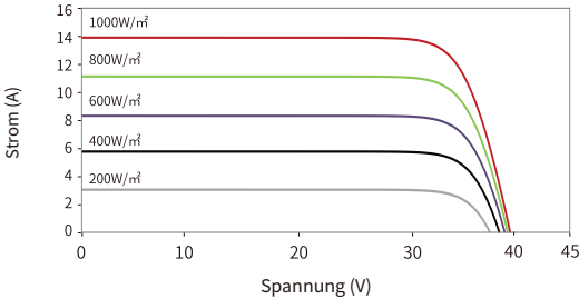
Strom-Spannungs-Kurven (54HL4R- (V) 450W)
